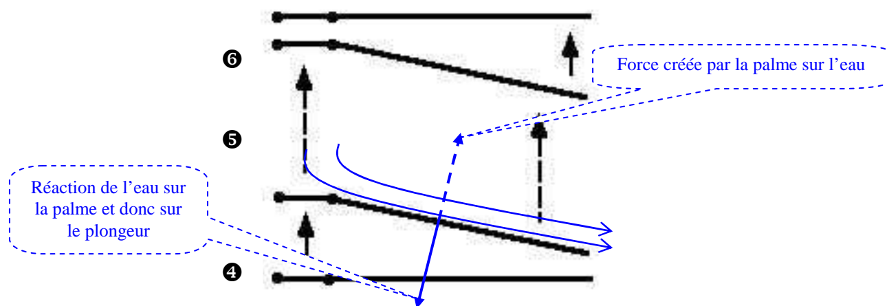
Figure 7.7 : Apparition de la force propulsive sur une palme lors de la phase de remontée (schéma extrait du site http://www.nageavecpalmes-ffessm.com et modifié par l'auteur).
