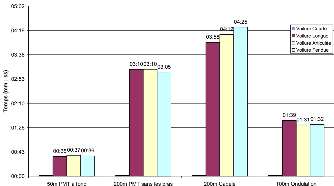
Figure 4.11 : Palmage type « du genou » - Résultats des tests
