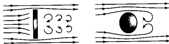
Figure 3.7 : Mise en évidence de la différence de traînée de pression entre une plaque plane et un cylindre (extrait de [Guyon et al. ; 2001])
